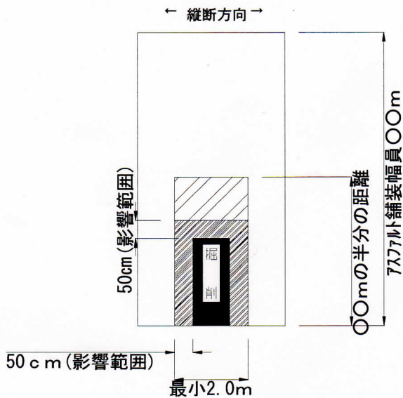
センターラインがない場合 (アスファルト舗装幅員が4m以上の道路) (半幅本復旧)
