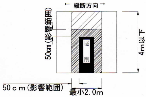
センターラインがない場合 (アスファルト舗装幅員が4m以下の道路) (全幅本復旧)
