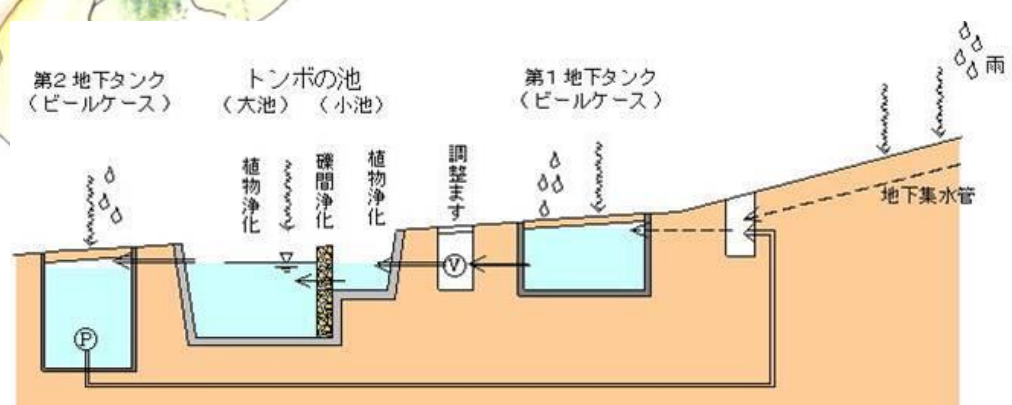
「トンボの池」の雨水循環システム
