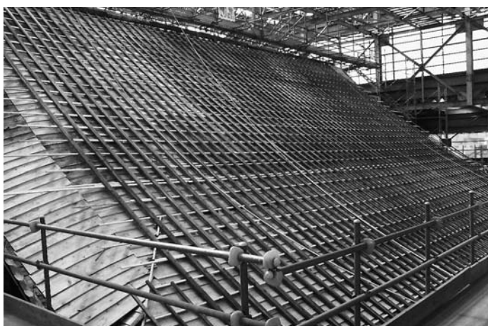
新瓦を葺く直前の本堂背面（空葺き工法）
