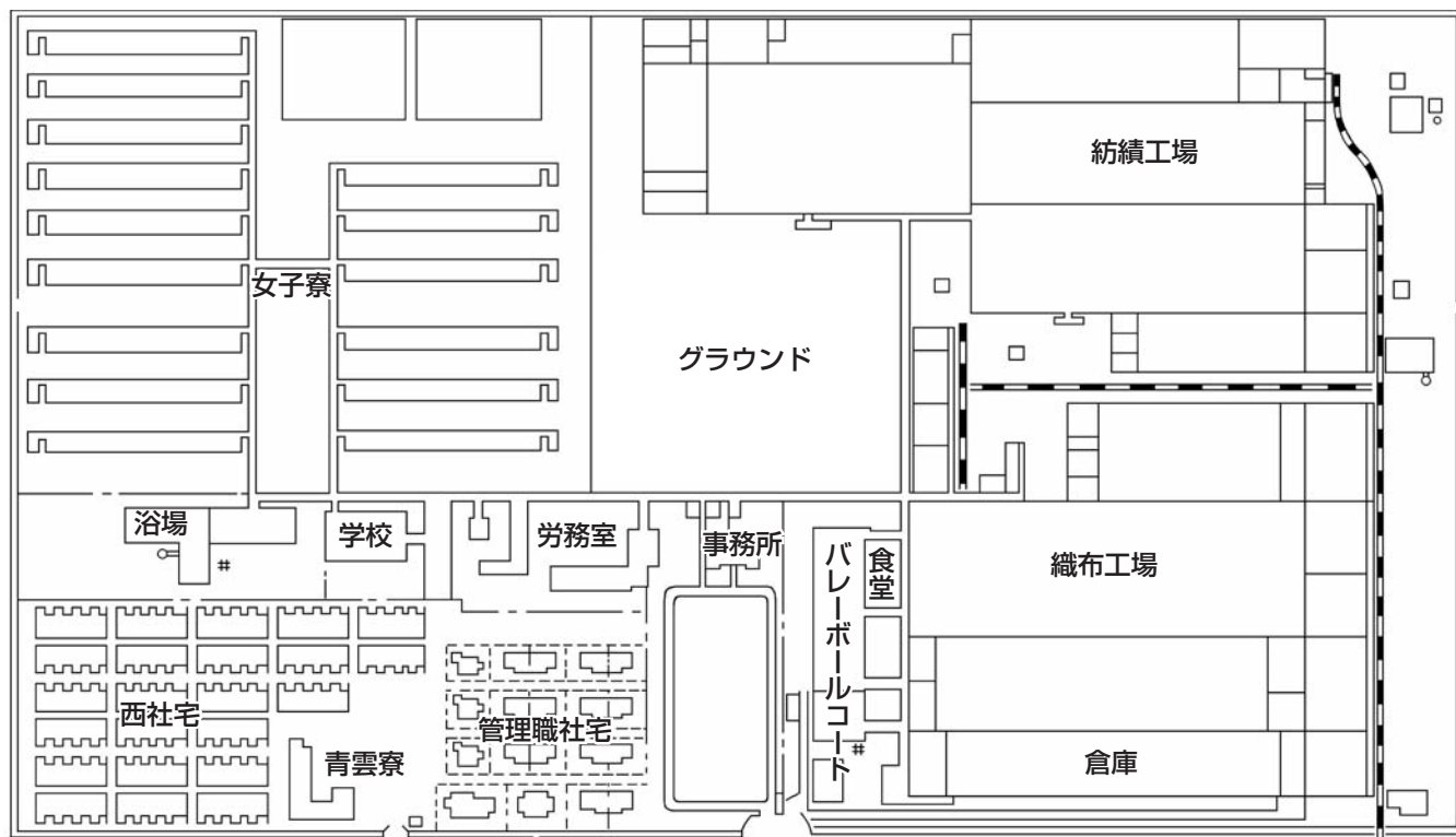
大日本紡績株式会社貝塚工場平面図（建築当初） ※本図は、ユニチカ記念館所蔵「自昭和十年六月 至十二年五月 雑書綴 第二號」所収の大日本紡績株式会社貝塚工場平面図（昭和10年5月当時）を下図にしています。
