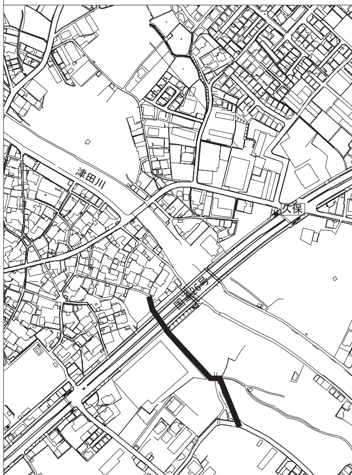
3. 小瀬処理分区污水管布設工事第27工区
