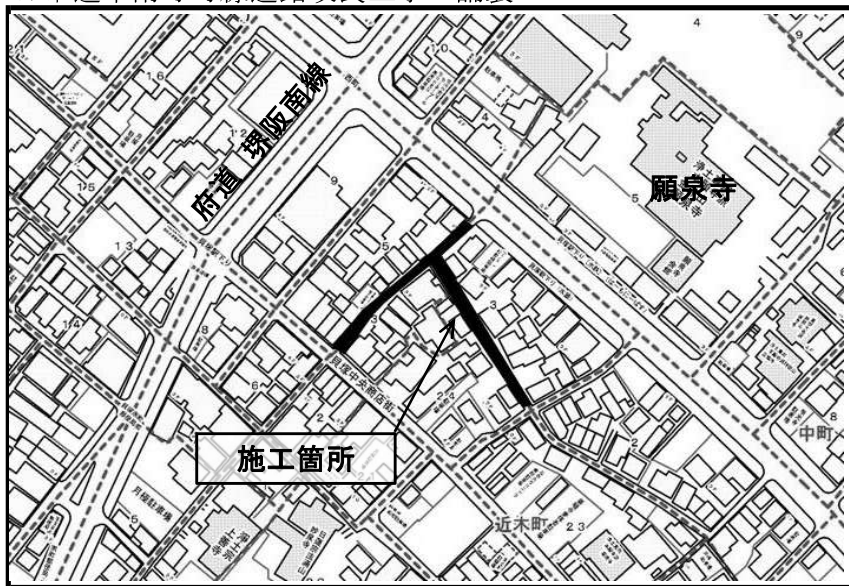
5. 市道中南寺町線道路改良工事・舗装
