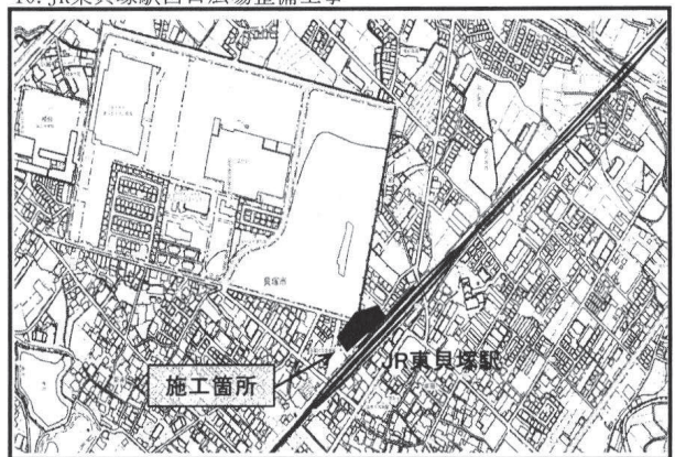
10. JR東貝塚駅西口広場整備工事
