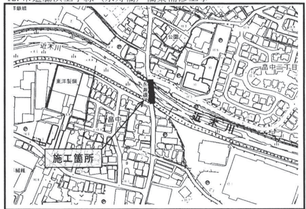
12. 市道臨浜王子線(永寿橋)橋梁補修工事
