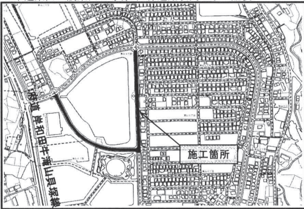
1. 市道東山丘陵東西1号線外1線道路改良工事・舗装
