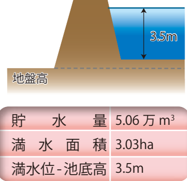
坂本池の断面イメージ（最大箇所）
