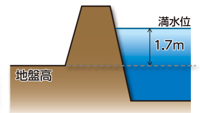
新井ノ池の断面イメージ(最大箇所)
