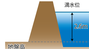
唐間池・堂の池の断面イメージ(最大箇所)
